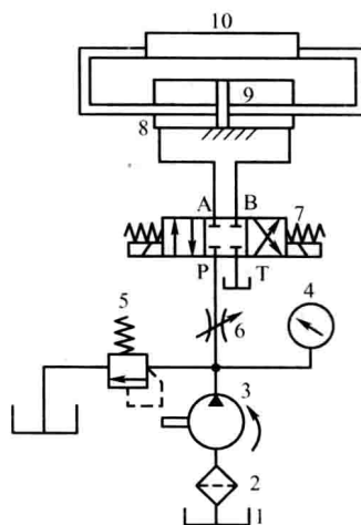
图 1-3 机床工作台的液压传动系统
