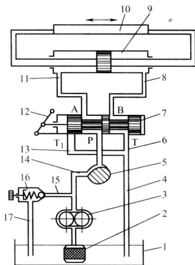
图 1-2 机床工作台液压系统原理结构图
