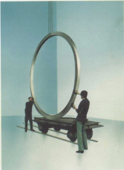
火箭大锻环
