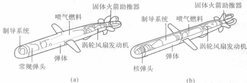
图1-2 美制“战斧”式巡航导弹的系统结构示意图
