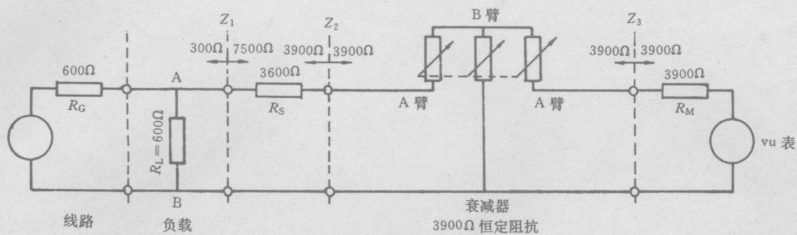
图 1 标准音量表的连接
