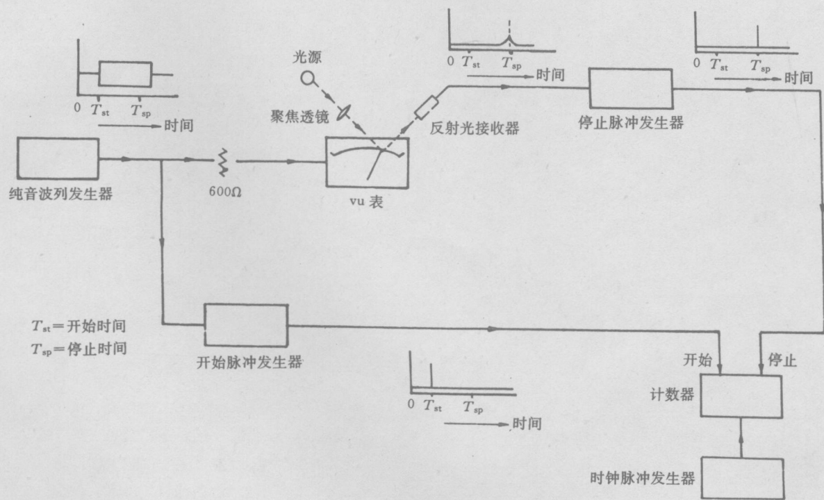
图 2 测量标准音量表响应时间仪器的示意图
