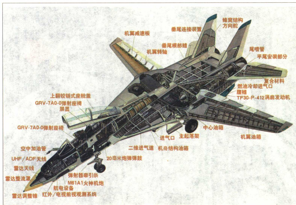
■F-14A“雄猫”战斗机局部剖视图。
