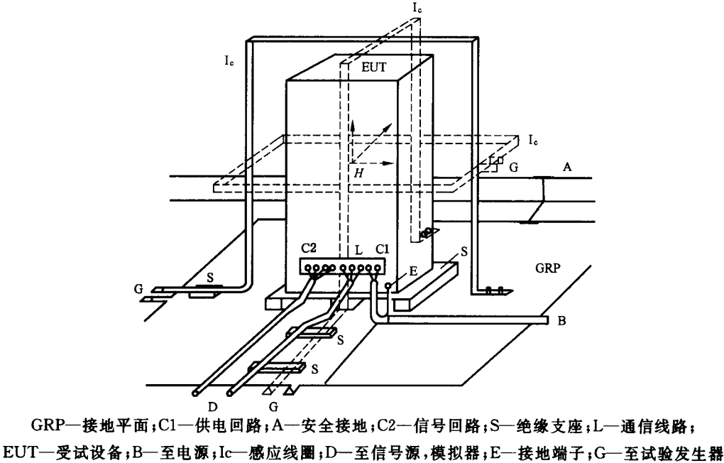
图 4 立式设备的试验布置
