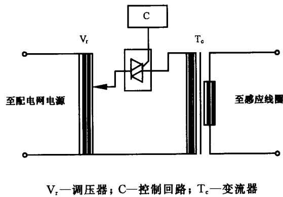
图 2 工频磁场试验发生器的原理图
