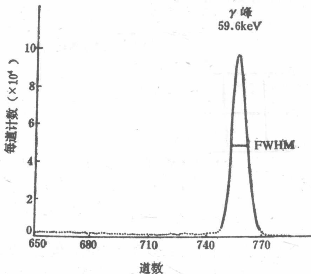
图3 ^{241}\text{Am} 的 59.6\text{keV} \gamma 峰
