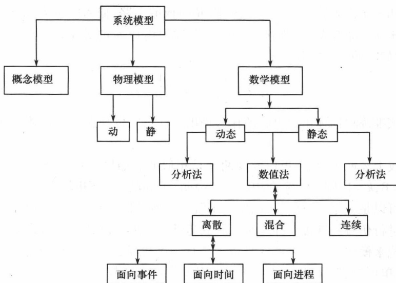
图 1-1 模型的分类
