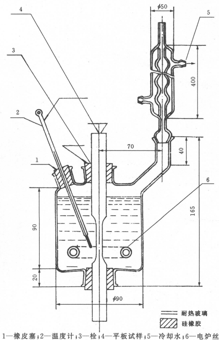
图 A2 恒负荷拉伸试验容器
