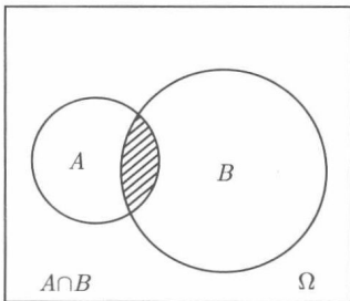
图 1-2 事件的交
