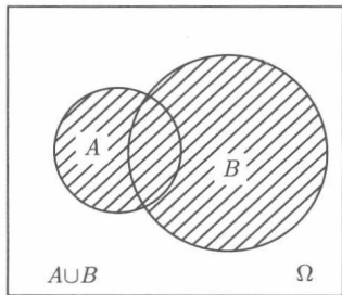
图 1-1 事件的并
