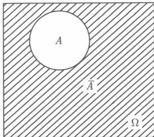
图 1-6 对立事件
