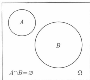
图 1-5 互不相容
