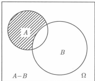
图 1-3 事件的差
