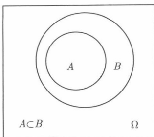
图 1-4 包含关系
