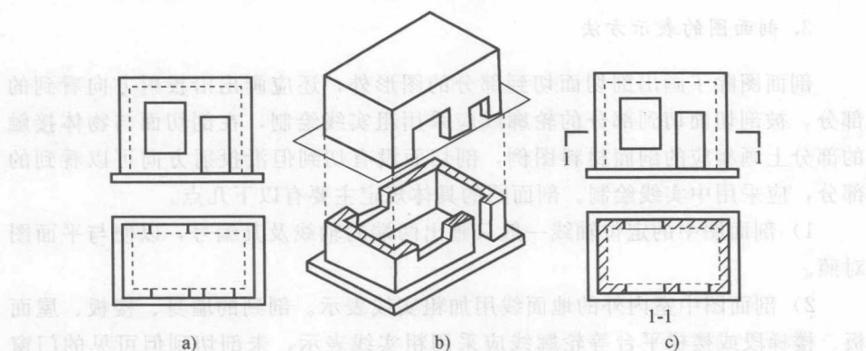
图 1-12 全剖图
