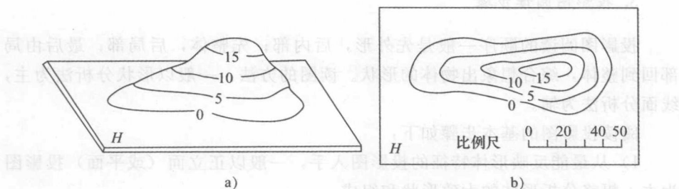
图 1-10 标高投影图
