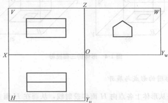
图 1-6 投影面展开图
