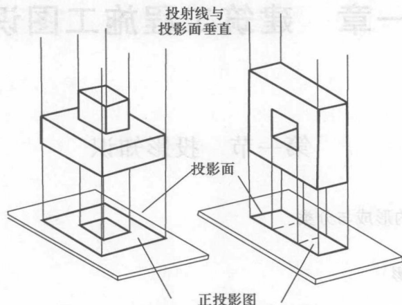
图 1-2 正投影图
