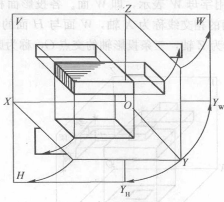
图 1-5 三个投影面的展开
