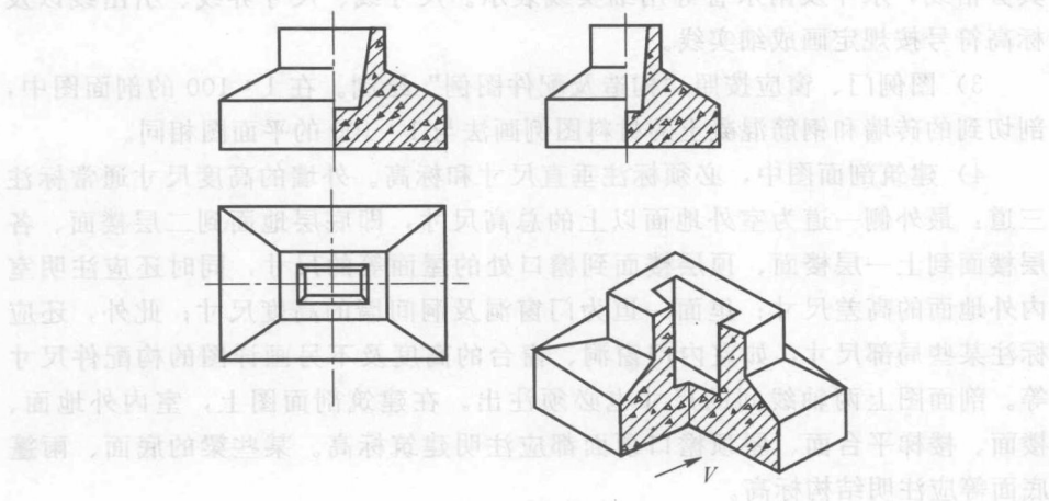
图 1-13 半剖图
