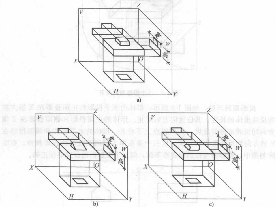
图 1-4 形体的三面投影
