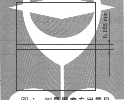
图 1 测量厚度专用量具
