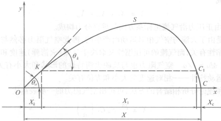
图 1.1 弹道
