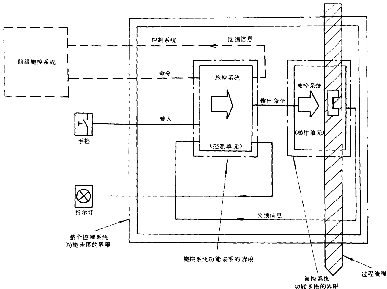
图 1 控制系统划分示例
