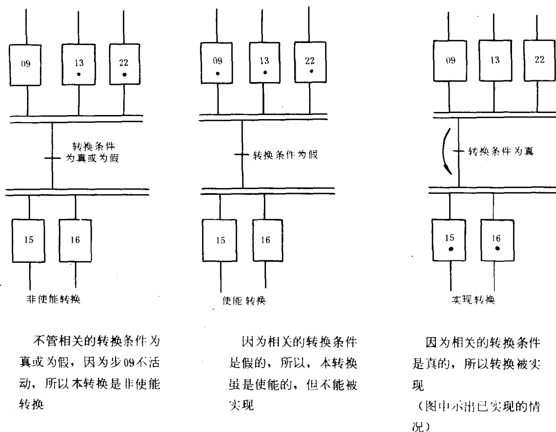
图 5 由几个前级步引起的使能和实现转换
