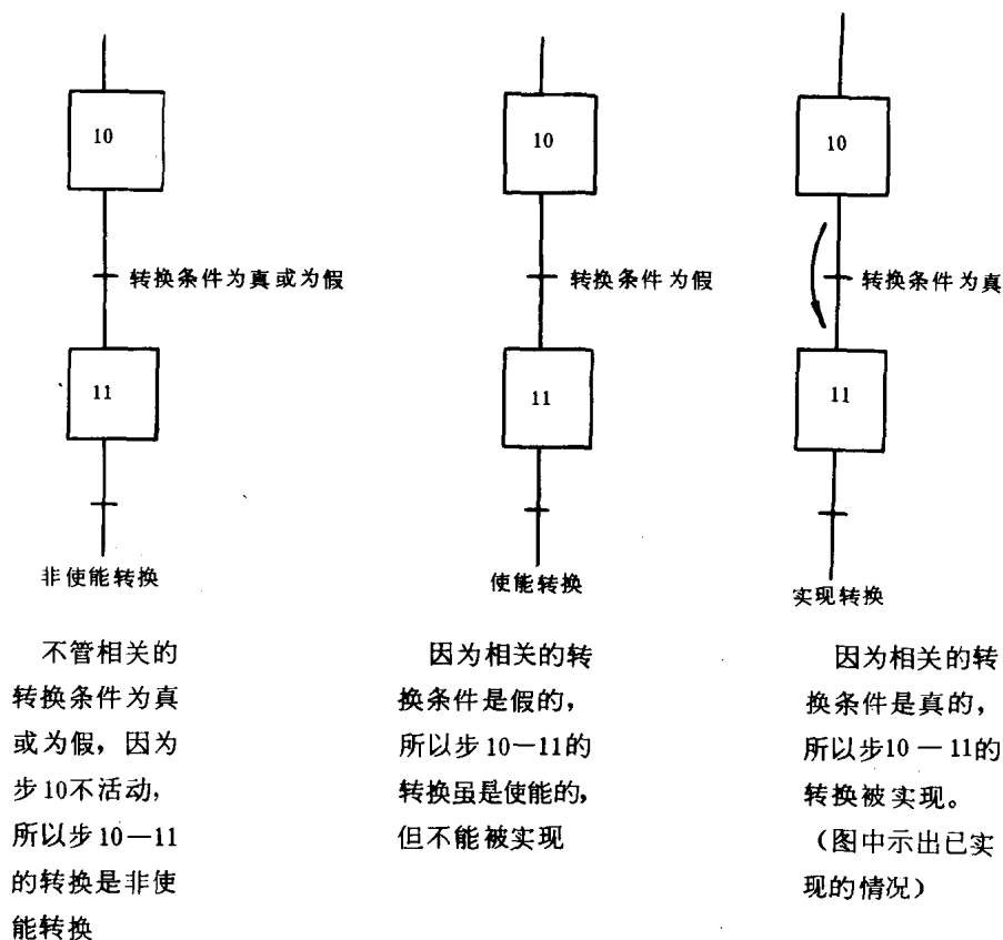
图 4 由一个前级步引起的使能和实现转换
