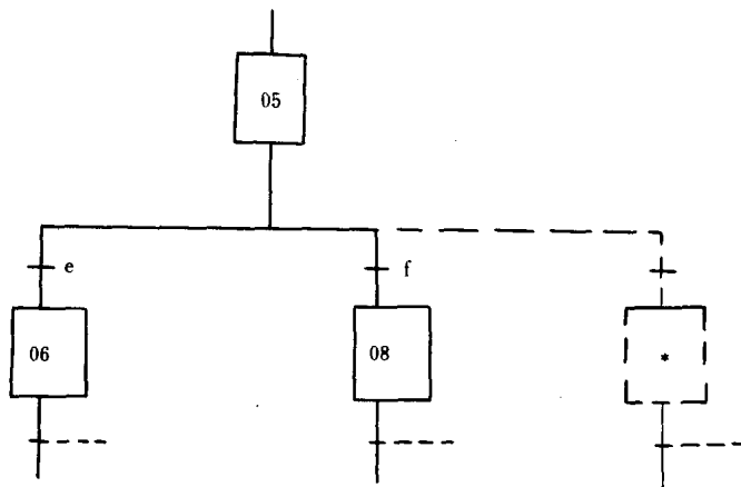
图 10 选择序列的开始示例
