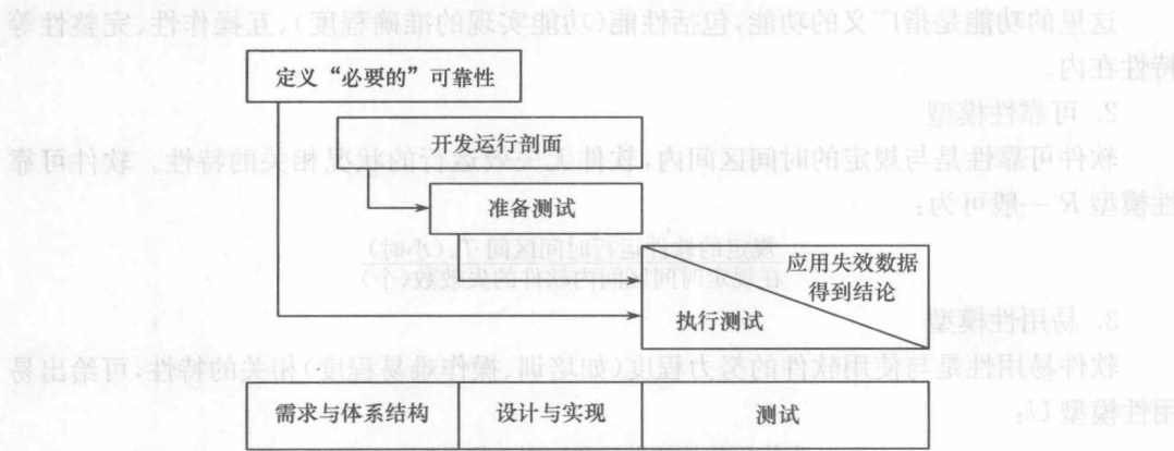
图 1.3 软件可靠性工程过程框架(Musa) [2]
