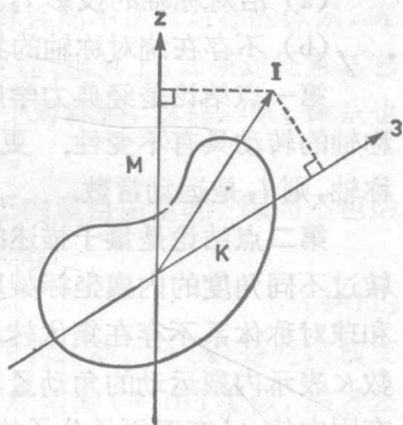
图 4-1 描述三维转动的角动量子数 z 轴属于实验室坐标系, 而 3 轴是本体坐标系的轴。[比较第一卷第 81 页图 1A-1 中的 \mathcal{R} 和 \mathcal{R}' 坐标系。]
