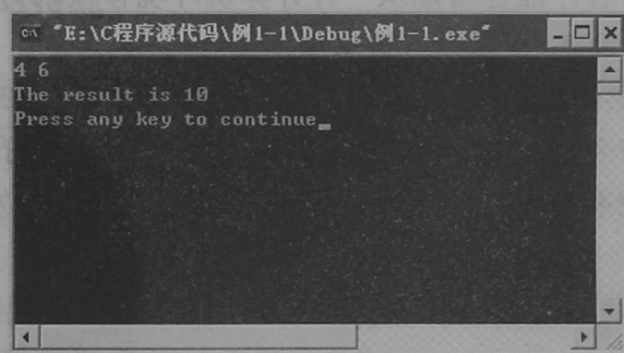
图 1-1 例 1-1 运行结果
