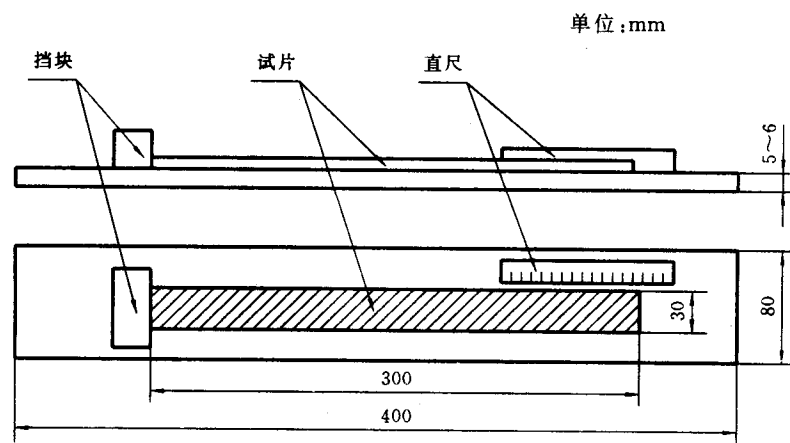
图 B1 测量方法示意图
