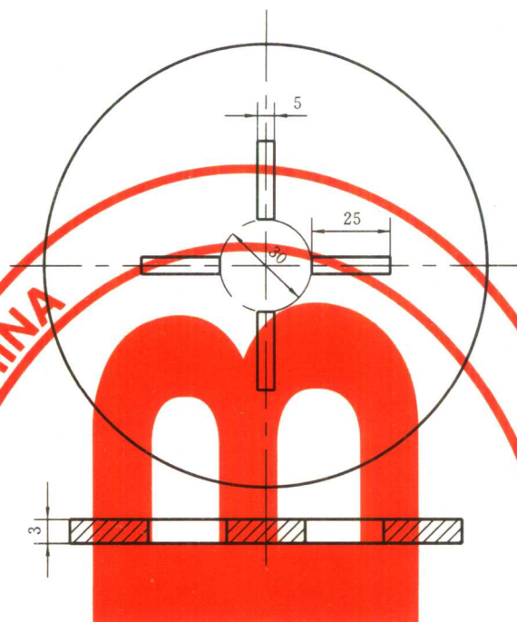
图3 透水仪压板示意图
