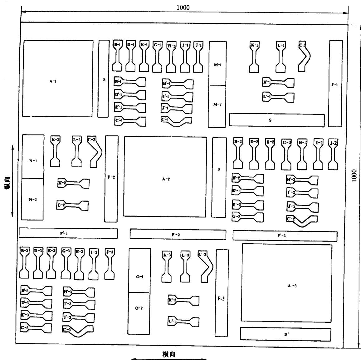
图 2 裁样示意图
