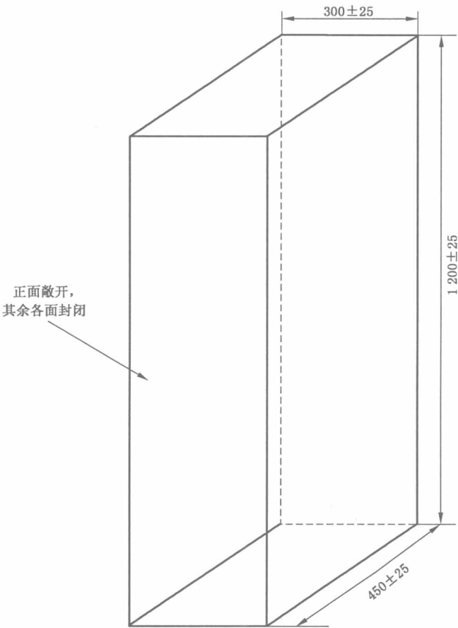
图 1 试验设备——金属罩
