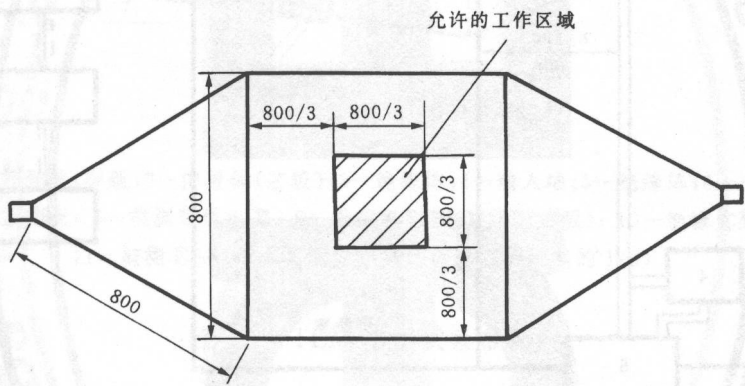
平面图
