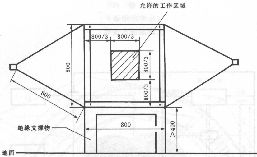
侧视图
