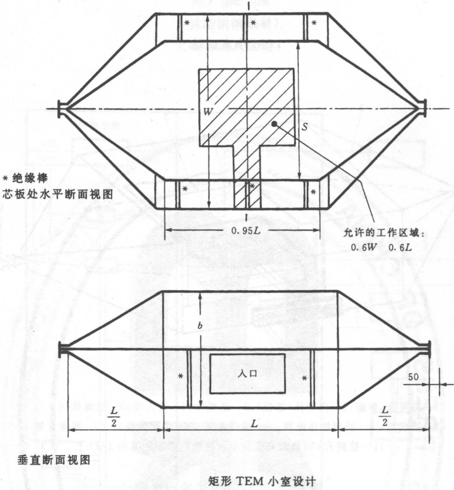
图 C2 TEM 小室尺寸
