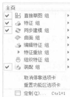
图 1-10 功能区菜单
