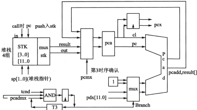
图 1-1 程序计数器运算控制结构框图
