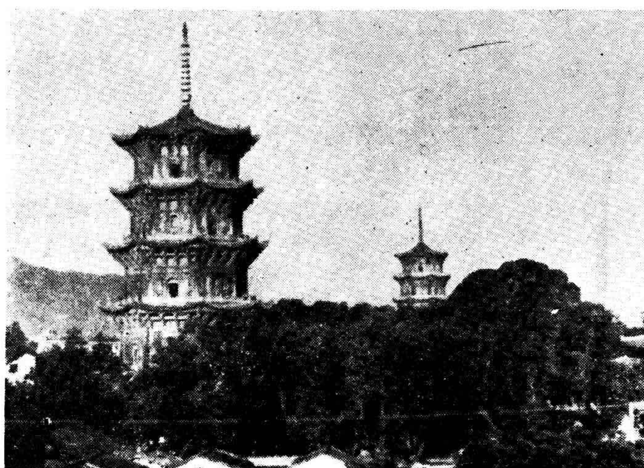
图29 泉州市开元寺双塔 南宋
