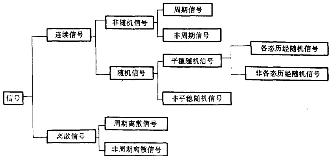
图1-2 信号分类
