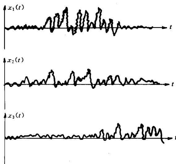
图1-1 不同语音所对应的不同声压波形
