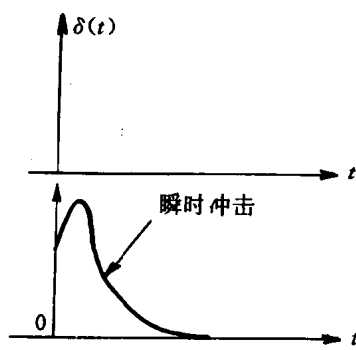
图1-6 瞬时冲击近似 \delta(t) 信号
