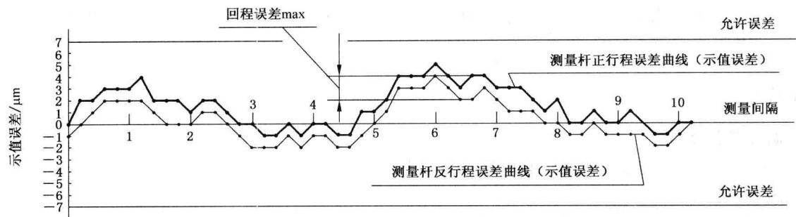
图 3 已设定零位的示值误差(曲线)示意图
