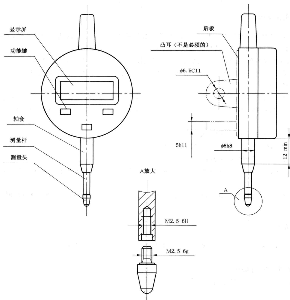
图 1 电子数显指示表的型式示意图
