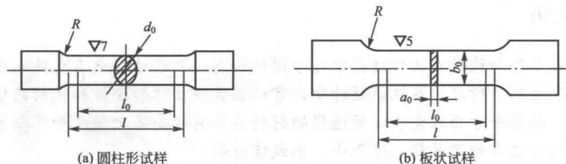
图 1.2 拉伸试样的形状
