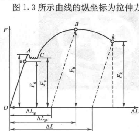
图 1.3 退火低碳钢拉伸力-伸长曲线
