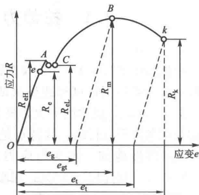
图 1.4 退火低碳钢应力-应变曲线
