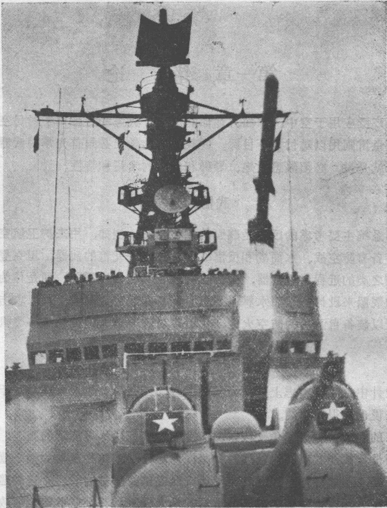
图1-1 这张照片说明了现代海军武器在战术上和技术上的紧密配合情况。照片中在舰炮的上方是正在发射出去的火箭助飞鱼雷。射击控制和搜索雷达高耸于上层建筑 and 主桅上
