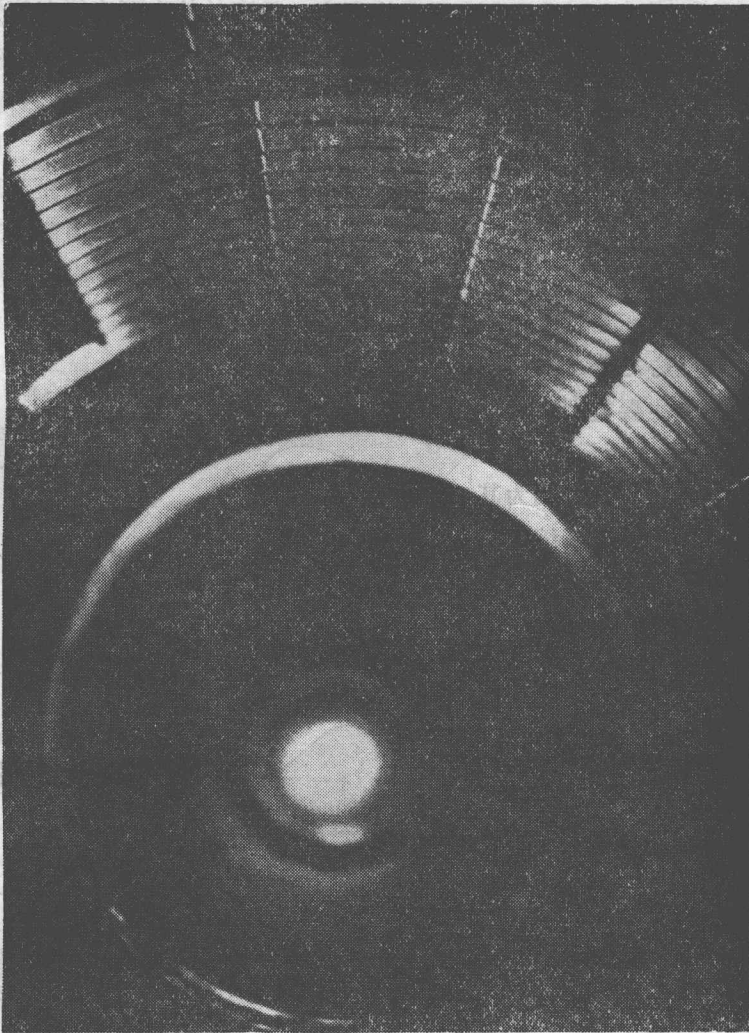
图2-1 内弹道学是研究从炮尾装进火药和炮弹，关闭炮门时起，直至炮弹离开炮口时为止所发生的情况
