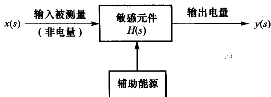
图 0-5 辅助能源型传感器
