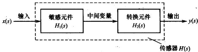
图 0-10 无转换电路
