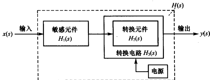
图 0-11 有转换电路
