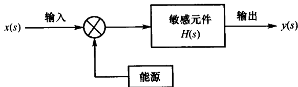
图 0-6 能量控制型传感器
