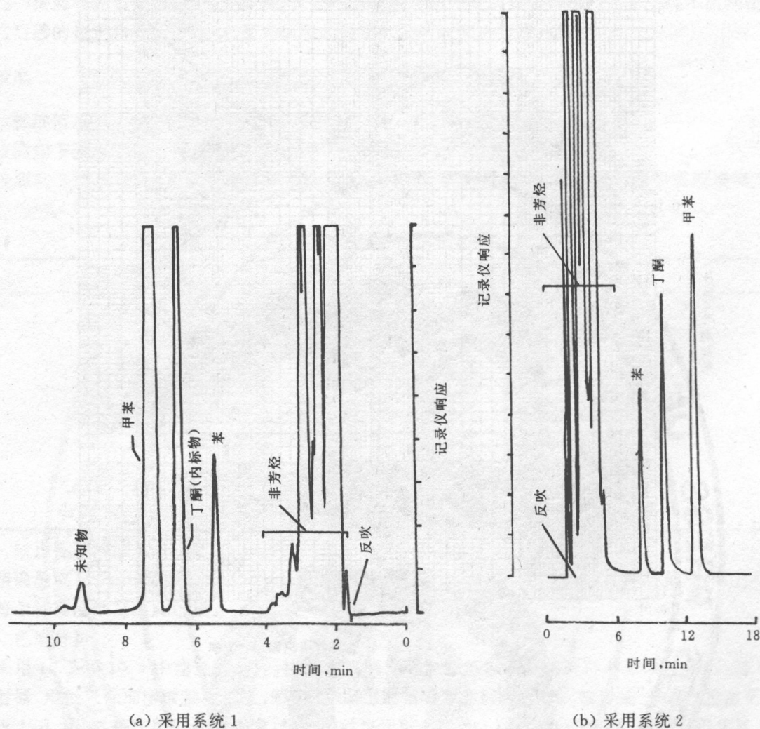
图 4 典型的气相色谱图
