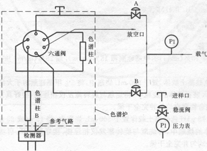
图 1 色谱系统连接示意图
