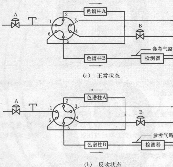
图 2 色谱气路系统示意图
