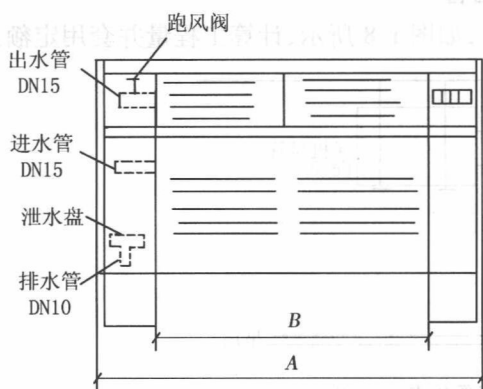
图 1-9 风机盘管示意图
