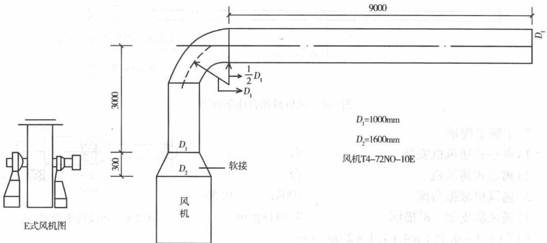
图 1-6 风机送风示意图
