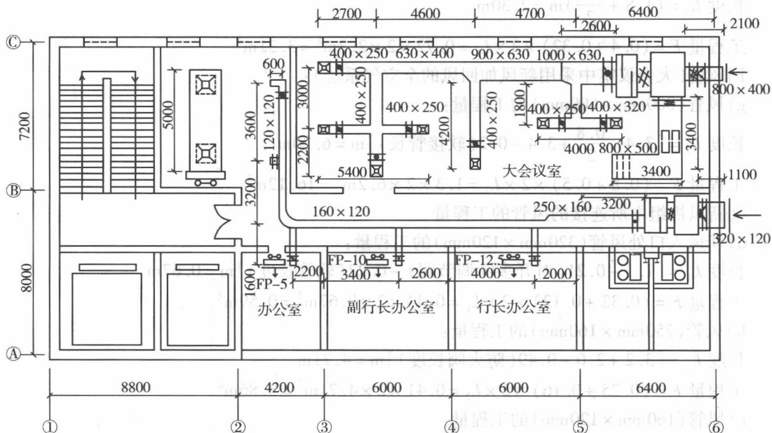
图1-11 送风平面图
