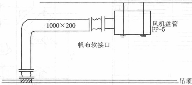
图 1-8 风机盘管安装示意图
