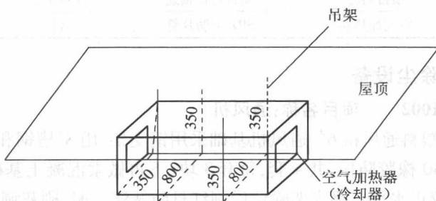
图 1-1 空气加热器安装示意图
