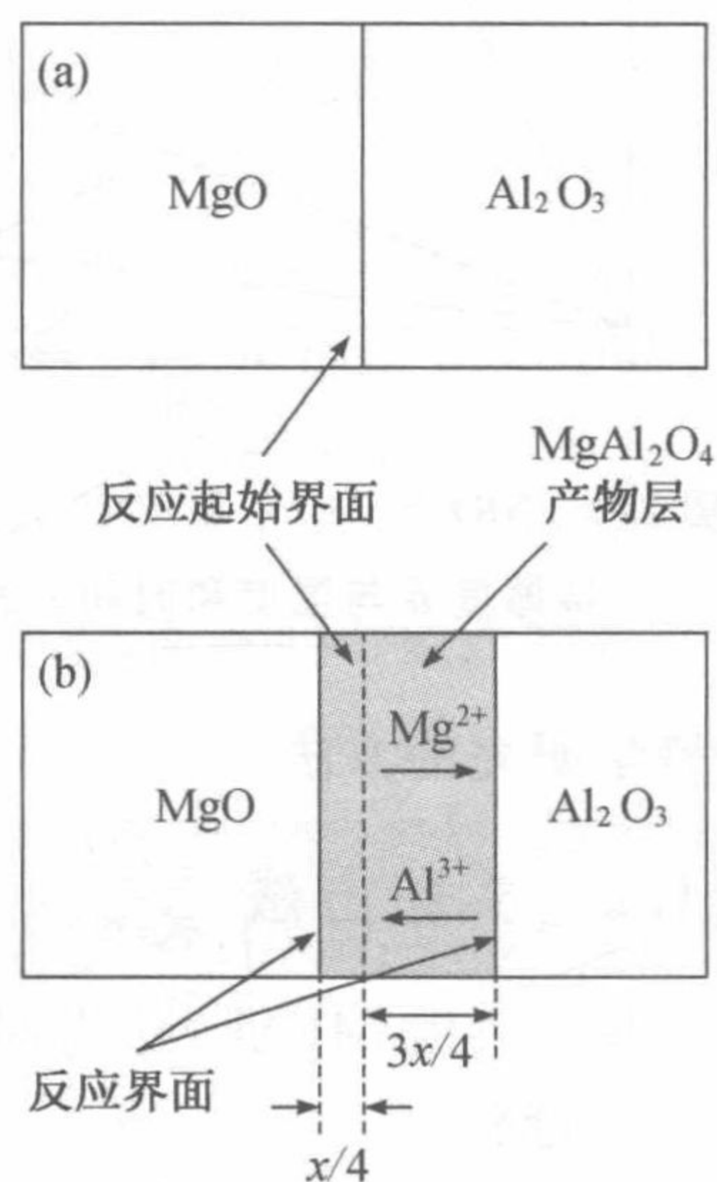
图 2.1 \text{MgO} 和 \text{Al}_2\text{O}_3 反应时相互紧密接触状态(a)和 \text{MgO} 与 \text{Al}_2\text{O}_3 中阳离子互扩散反应(b)示意图
