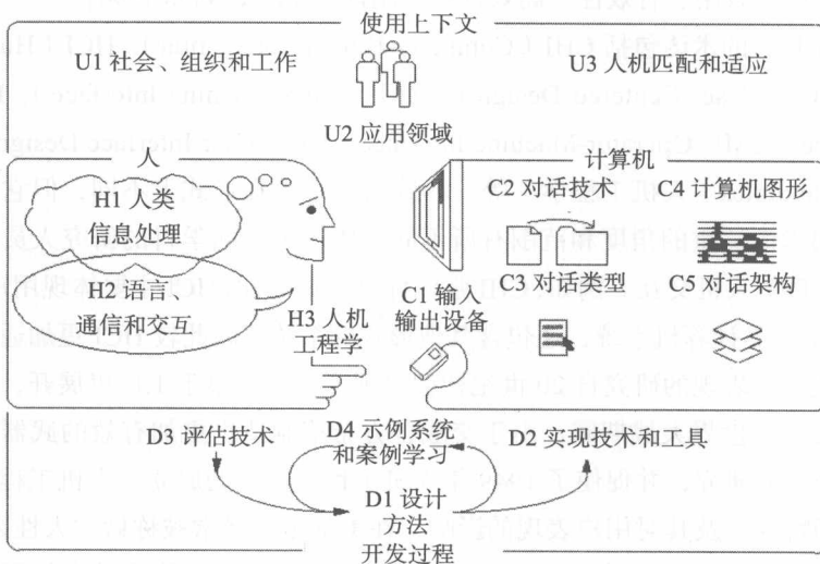
图 1-1 人机交互的研究内容
