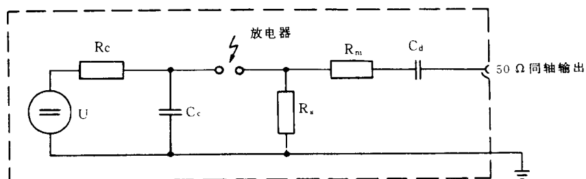
图 1 快速瞬变脉冲群发生器电路简图
