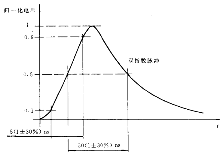
图 3 接 50 Ω 负载时单个脉冲的波形
