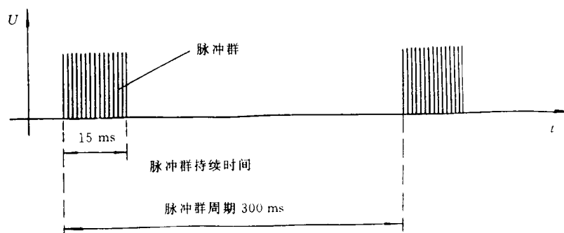
图 2 快速瞬变脉冲群概略图
