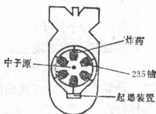
图 1—2 原子弹构造示意图
