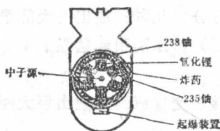
图 1—3 氢弹结构示意图
