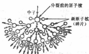
图 1—1 铀核裂变的链式反应示意图
