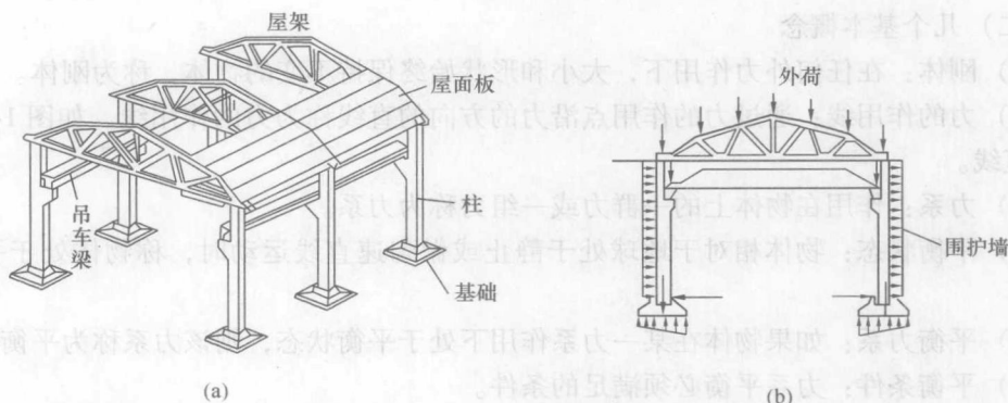
图 1-0-1 单层厂房的结构示意图
