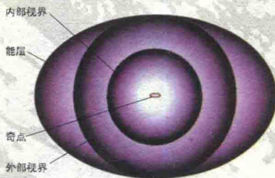
旋转的黑洞
