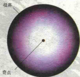
静止的黑洞
