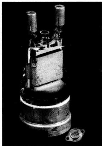
图 0-1 电子管与晶体管
