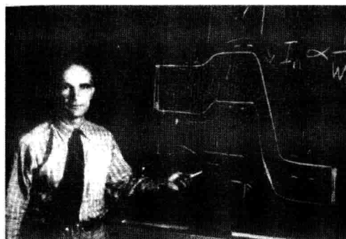
图0-4 肖克莱讲授半导体能带理论
