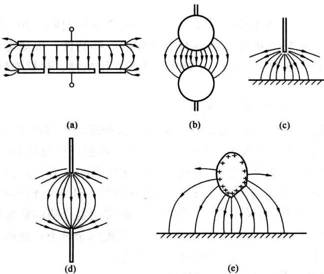
图 1-1 均匀电场与不均匀电场示意图
