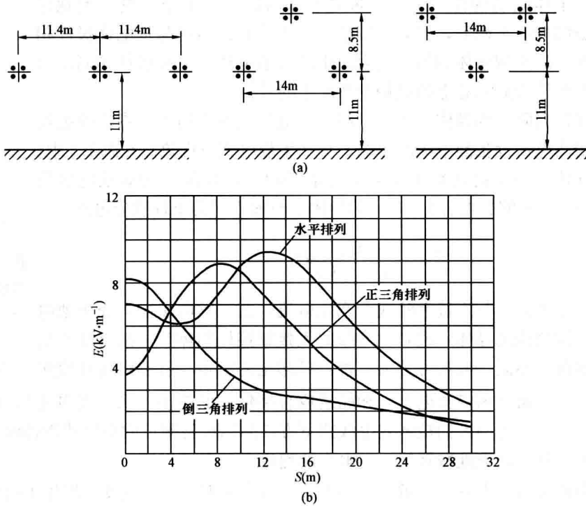
图 1-3 500kV 输电线路下方的工频电场
