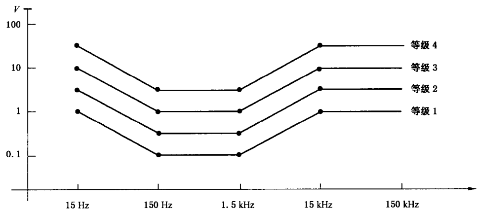
图 2 试验电压曲线
