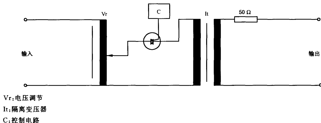
图 4 电源频率(16⅓ Hz、50 Hz 和 60 Hz)试验发生器准则示意图
