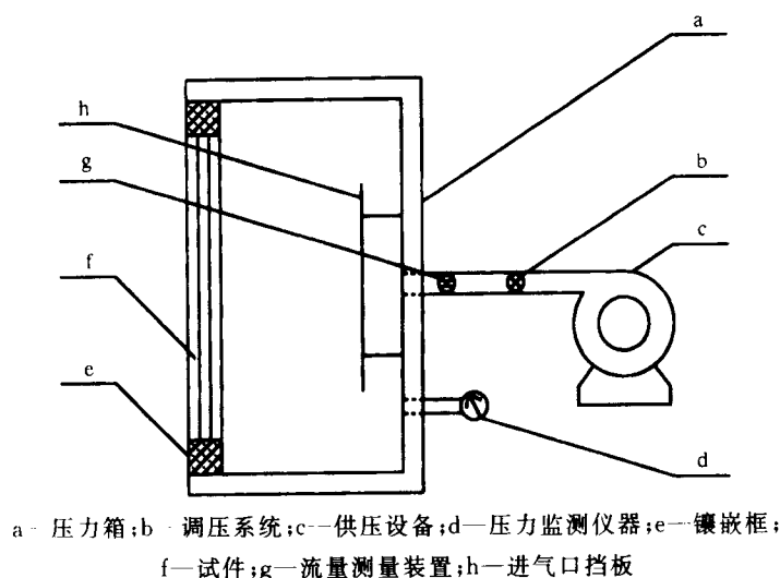
图 1 检测装置示意图
