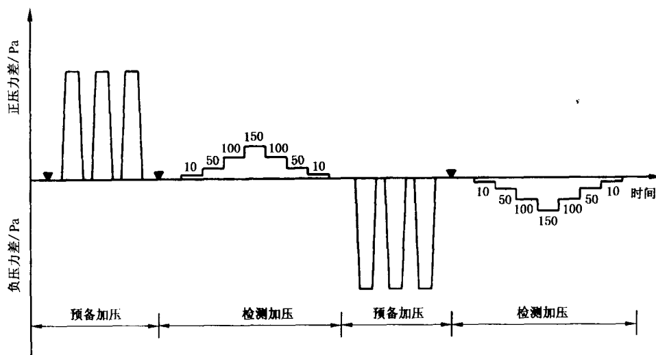
图 2 检测压差顺序图
