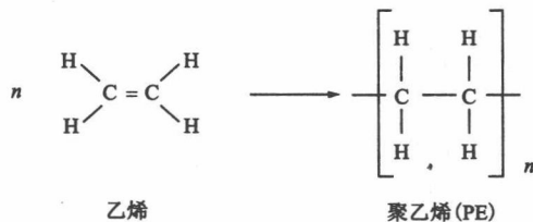
图 1-2 乙烯聚合反应示意
