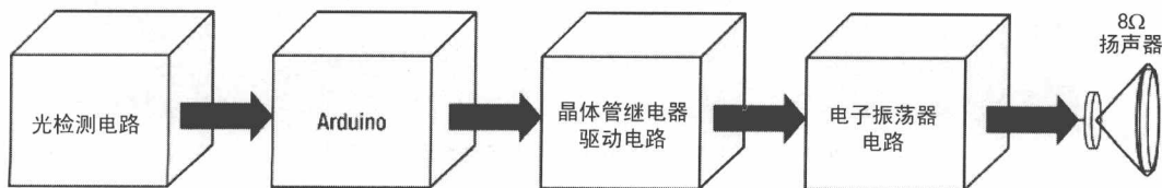
图 1-2 电子鸣鸟的系统方框图
