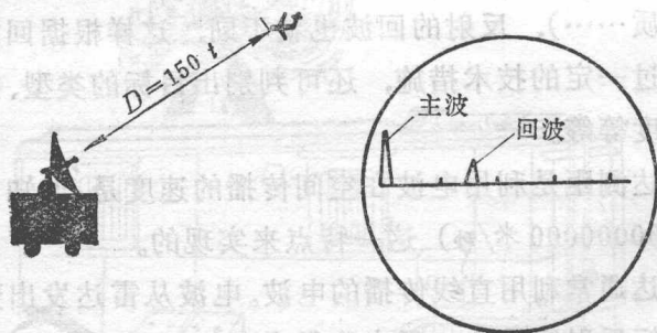
图2-2 测距原理示意图
