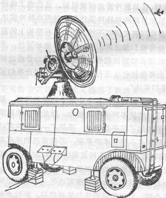
图2-1 圆锥扫描制炮瞄雷达战斗状态图
