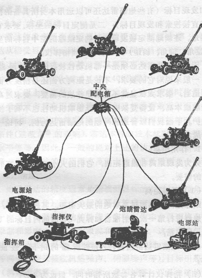
图1-1 地面防空火力系统示意图
