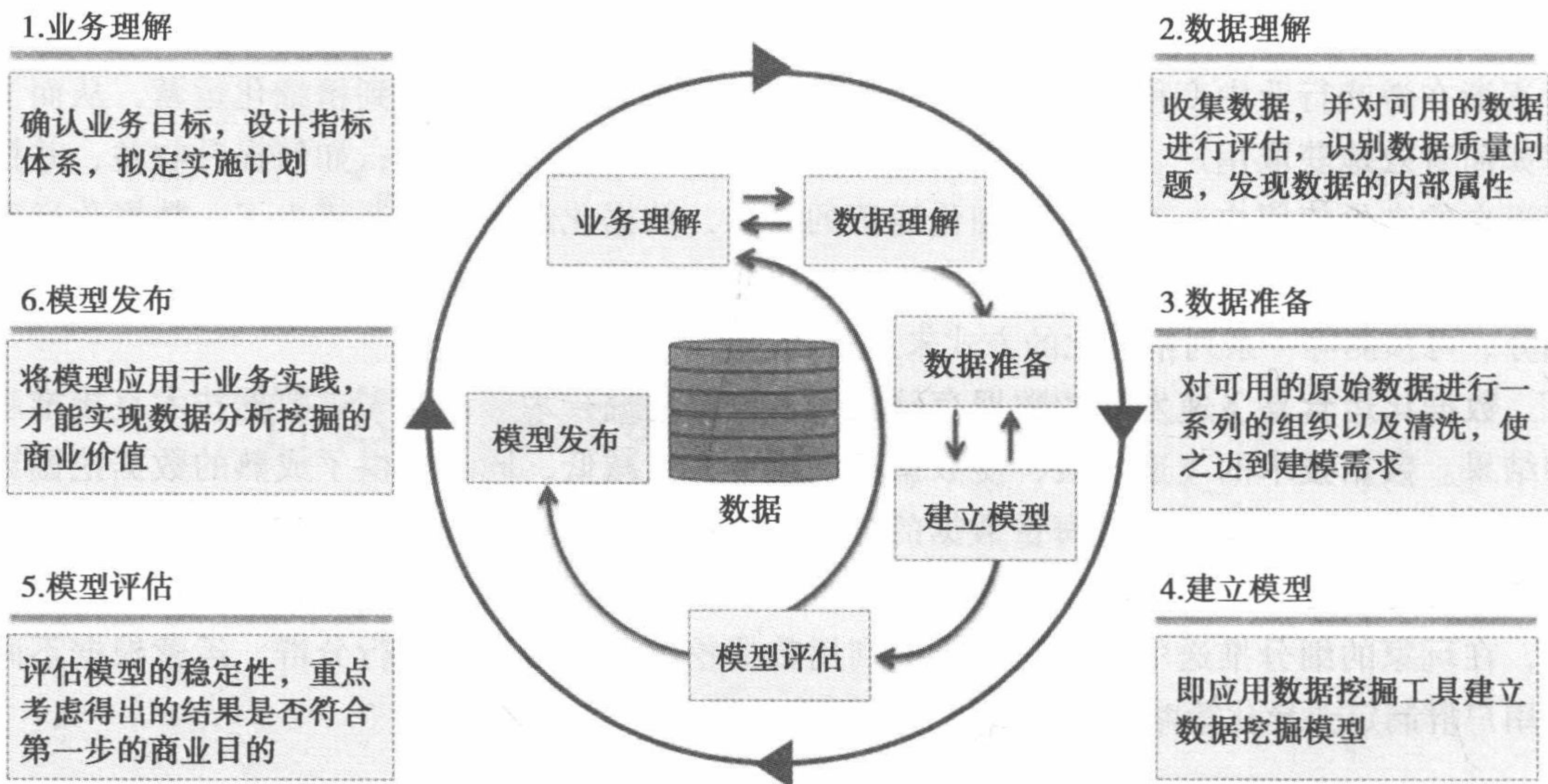
图 1-1 CRISP-DM 方法论示意图
