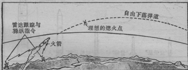
图1-3 指令制导
