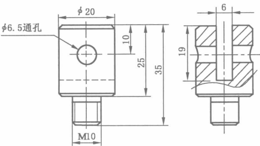
图 B.2 连接端头示意图
