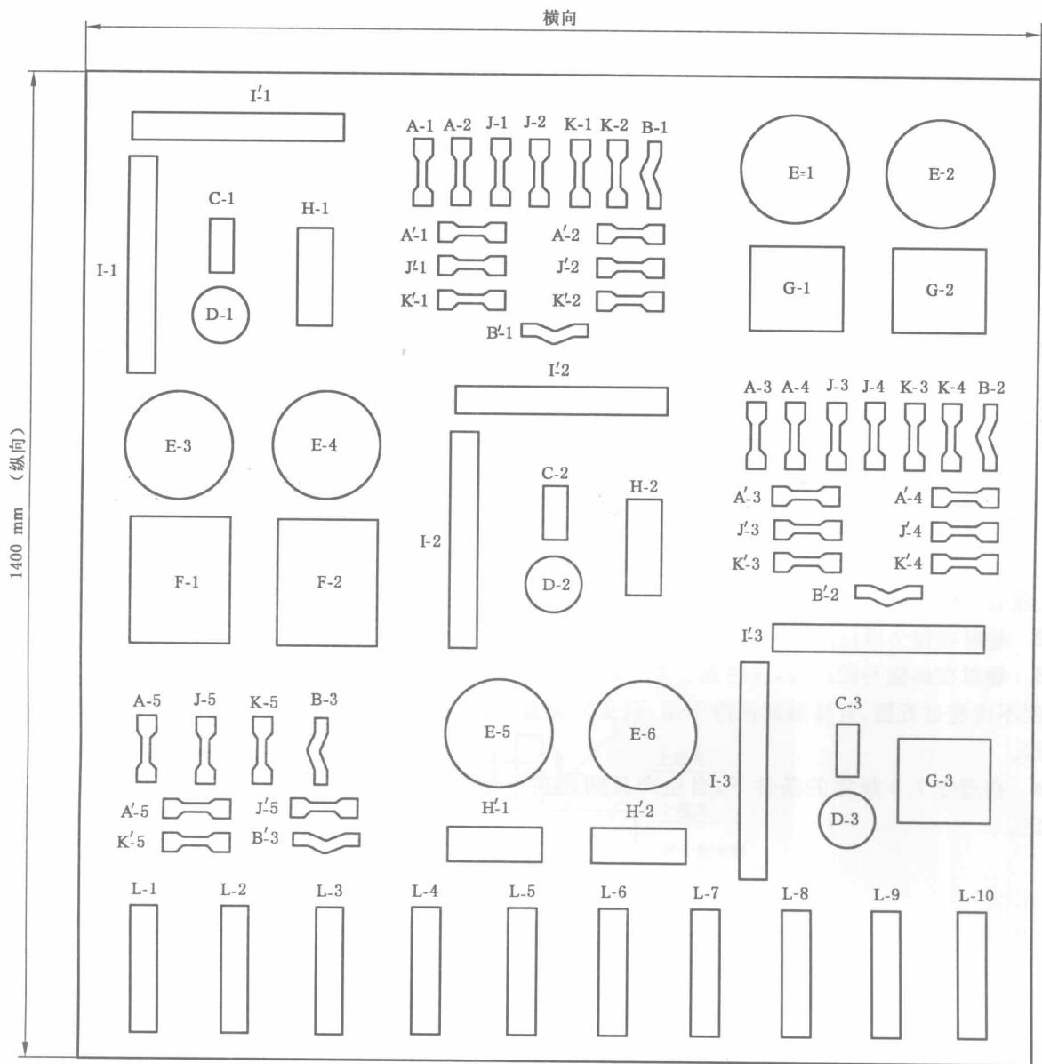
图 5 裁样示意图
