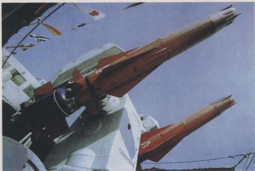
英国“海标枪”舰空导弹
