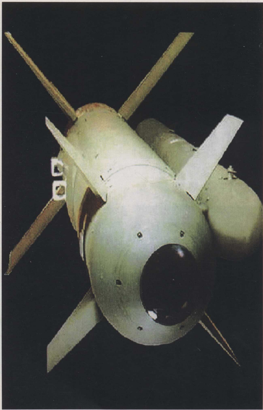
杀伤力最大的空地导弹——美国 AGM-130 空地导弹
