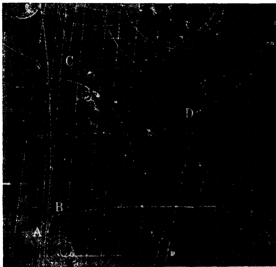
图 1.1 非常小的物体的前沿。气泡室中基本粒子的径迹。在一场亚微观领域的猛烈碰撞中，A 点处两个粒子毁灭，另三个粒子产生。碰撞空间延伸 10^{-16}\text{m} ，时间延续 10^{-23}\text{s} 。在 B、C、D 处有粒子相互作用的其它事件产生。本照片摄于 1964 年，帮助证实了新粒子 \Omega^- 的存在。 \Omega^- 留下从 A 到 B 的径迹。用于记录这些径迹的气泡室见图 3.10(b)。
