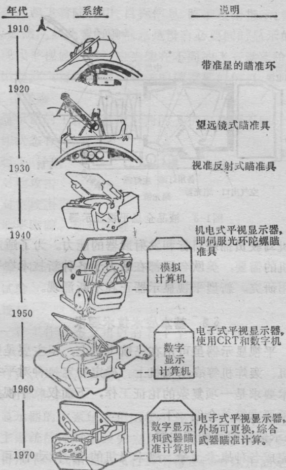
图1-2 平视显示器的发展过程
