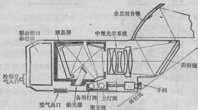
图1-3 液晶全息平视显示器
