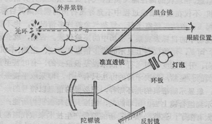
图1-1 瞄准具的显示方法
