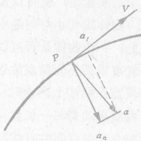
图 1—2 曲线运动的加速度
