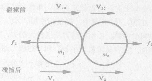
图 1-5 动量守恒定理
